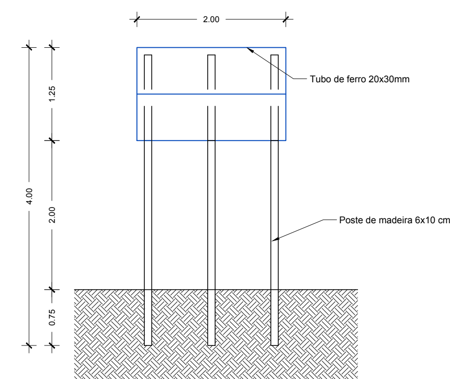
04 PLACA DA OBRA ESCALA 1:50
