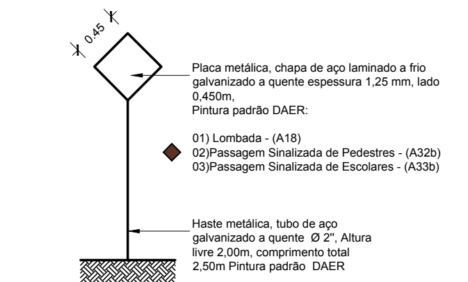
09 PLACAS DE TRÂNSITO - A18 ESCALA 1:50
