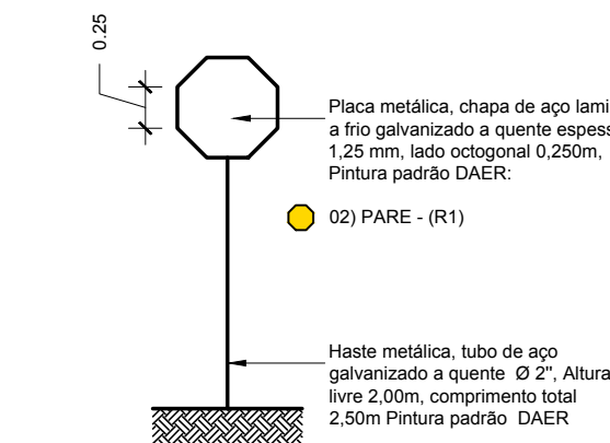
08 PLACAS DE TRÂNSITO - R1 ESCALA 1:50
